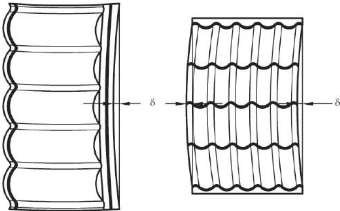
Рисунок 6 - Серповидность
